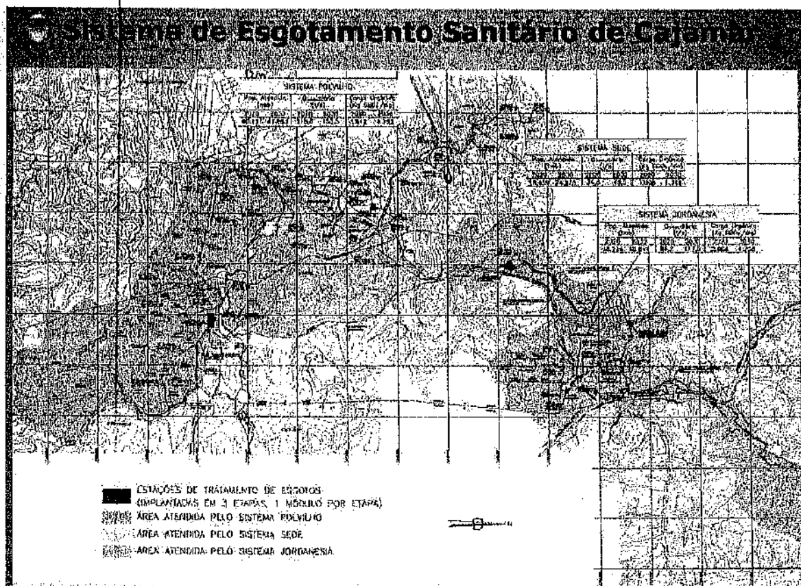
Figura 16 Esquema geral de esgotos de Cajamar
